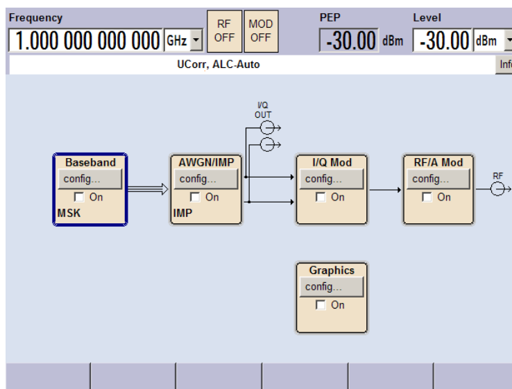
図 4-1: すべての機能を装備した R&S SMBV のブロック・ダイアグラム
