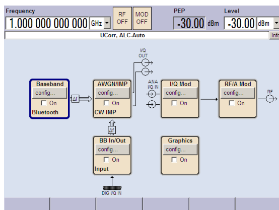
図 3-1: すべての機能を装備した R&S SMBV のブロック・ダイアグラム
