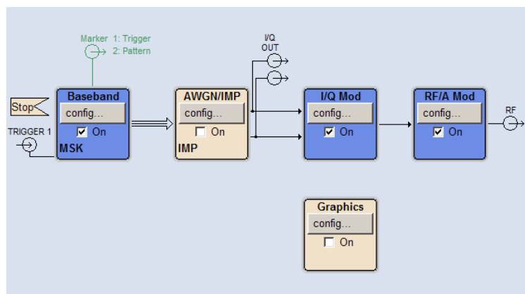
図 4-2: R&S SMBV のブロック・ダイアグラム
